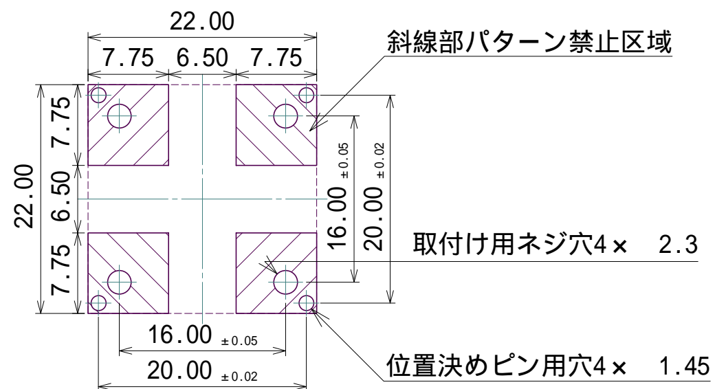
基板取付け参考図
